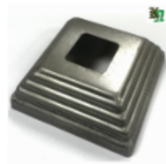
Основа балясины, арт. R10436.02 80х80х1мм, кв.25х25мм Вес: 0.075 кг Цена (за шт): 10 руб.
